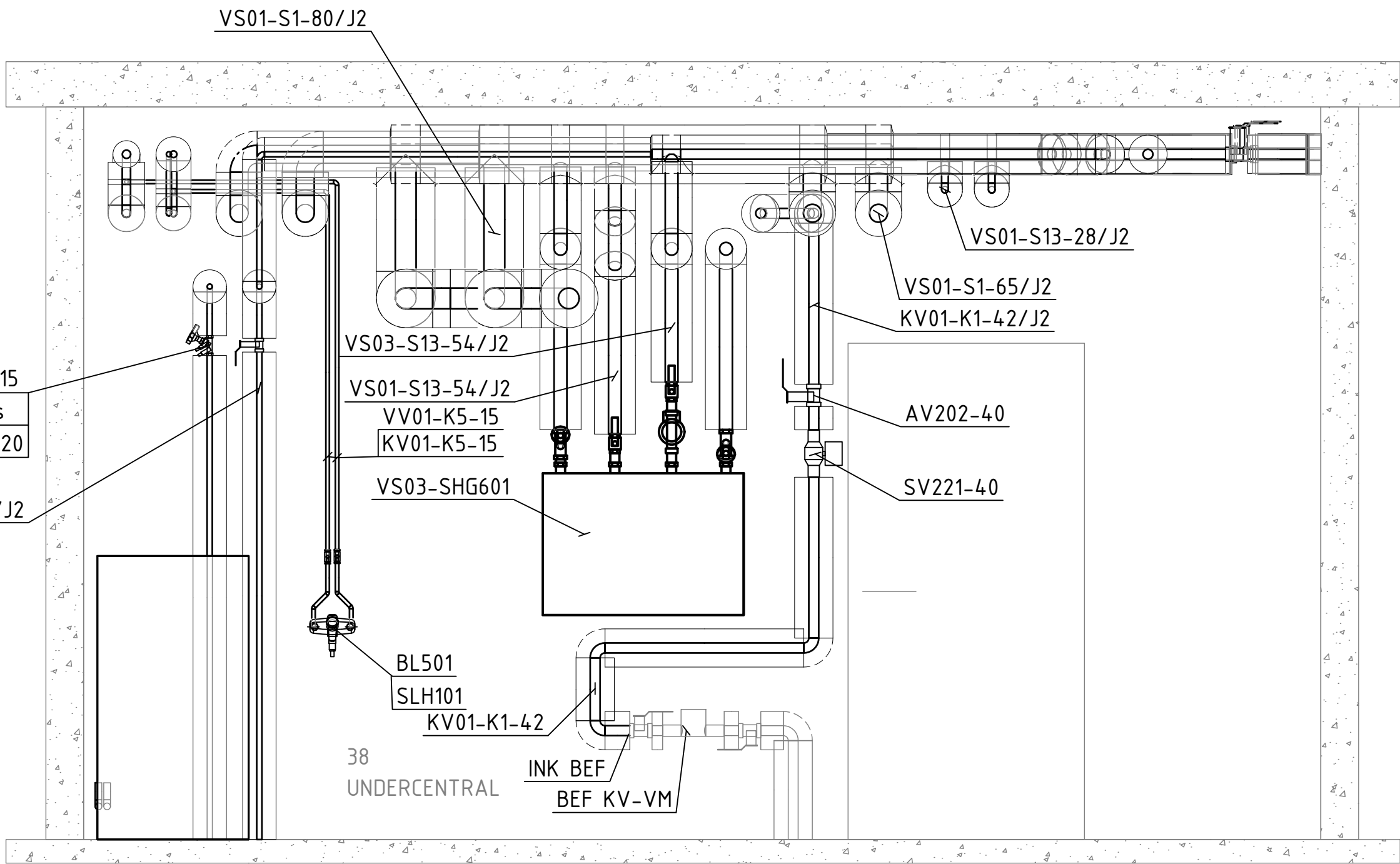
SEKTION 3 SKALA 1:20
