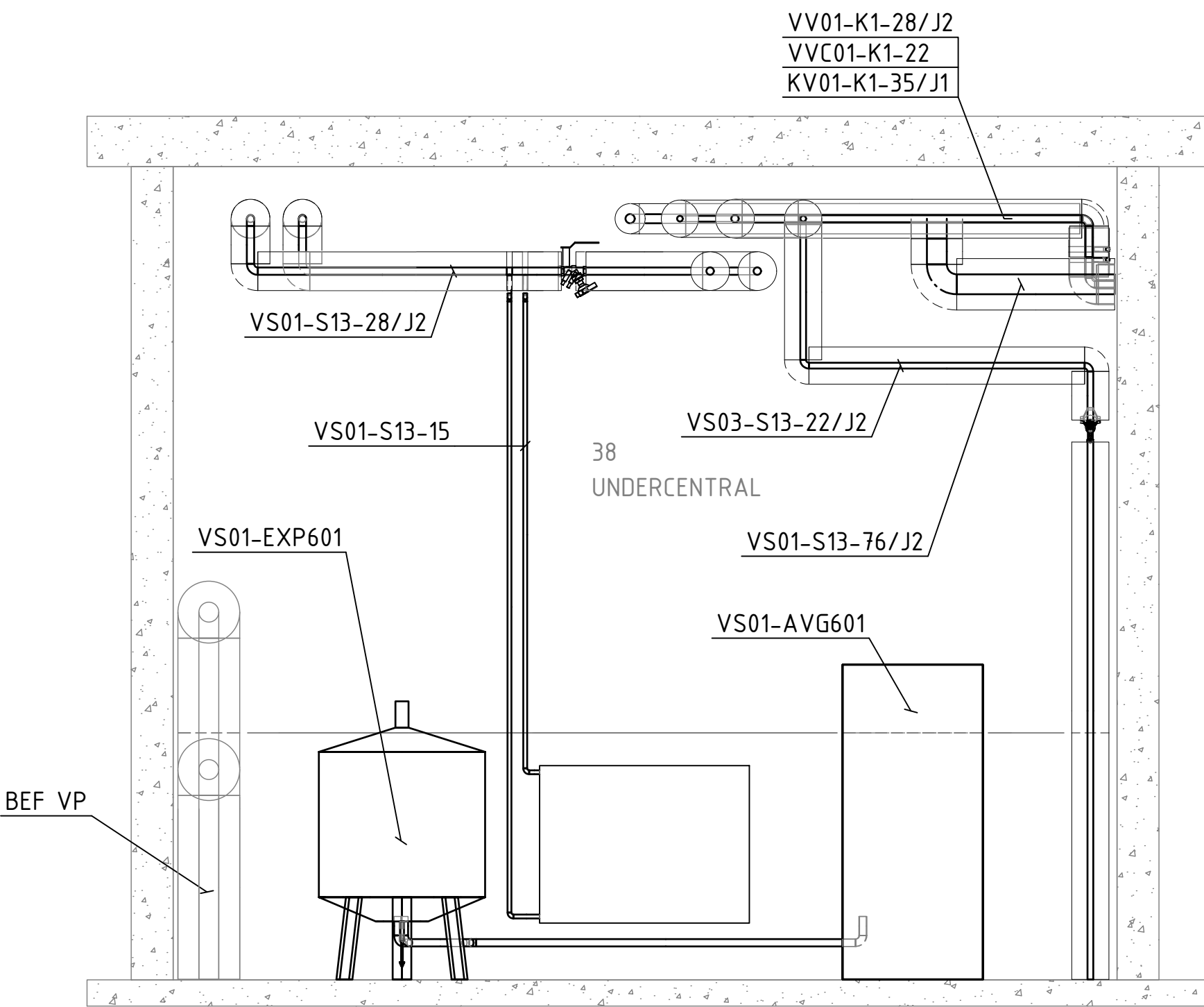
SEKTION 5 SKALA 1:20
