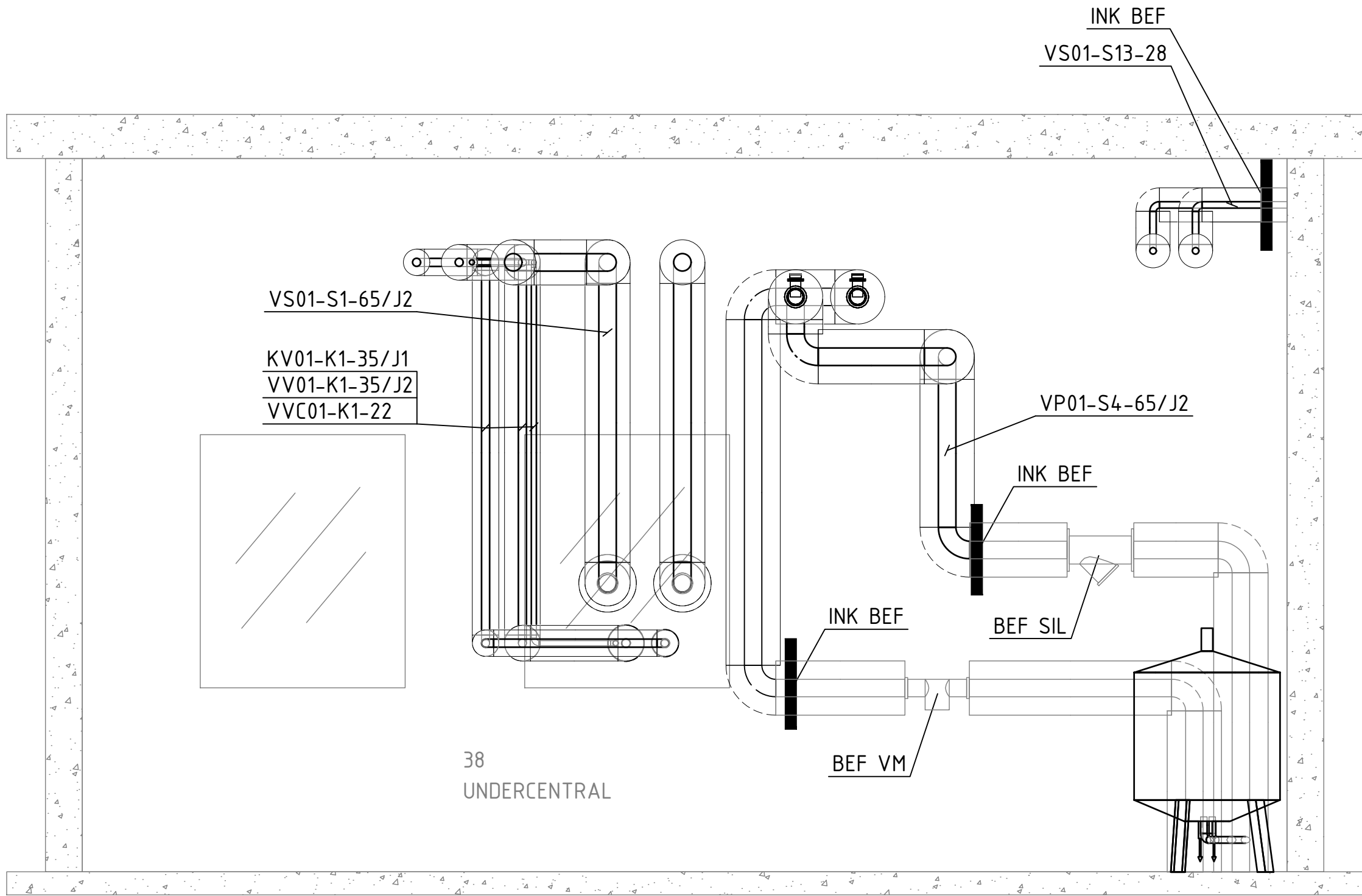
SEKTION 2 SKALA 1:20
