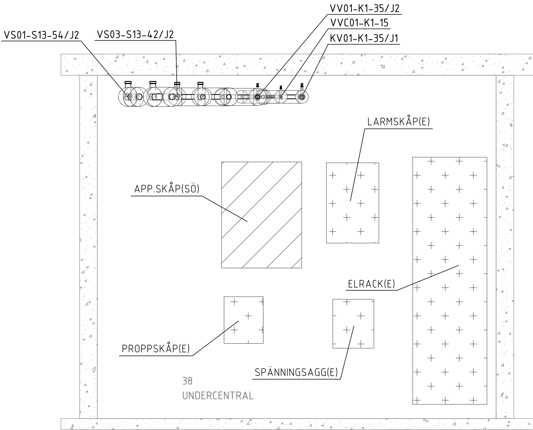
SEKTION 4 SKALA 1:20
